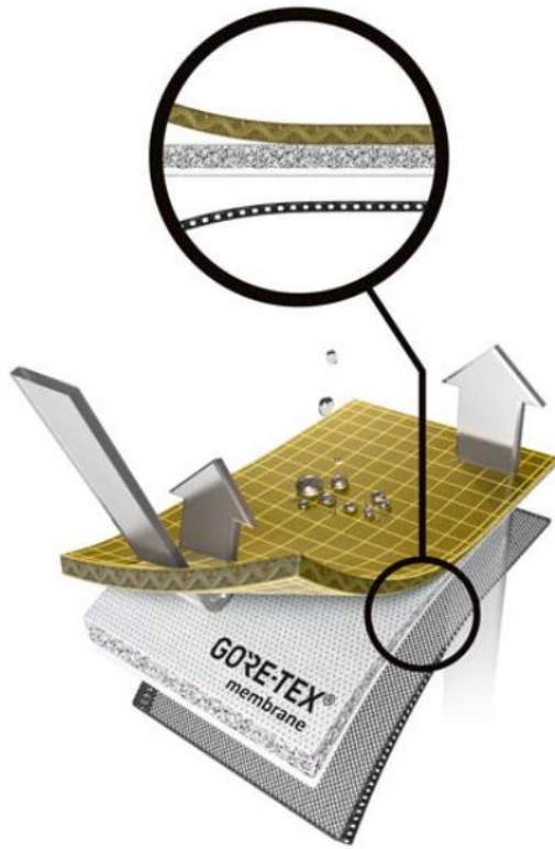
GORE-TEXメンブレンの片側にのみ生地を圧着したものが2レイヤー
