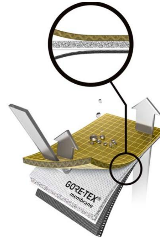
3つの層全てがGore社開発のため、防水透湿の最新技術が凝縮されています
